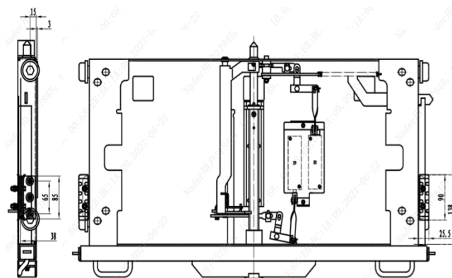
配柜宽 1000mm
