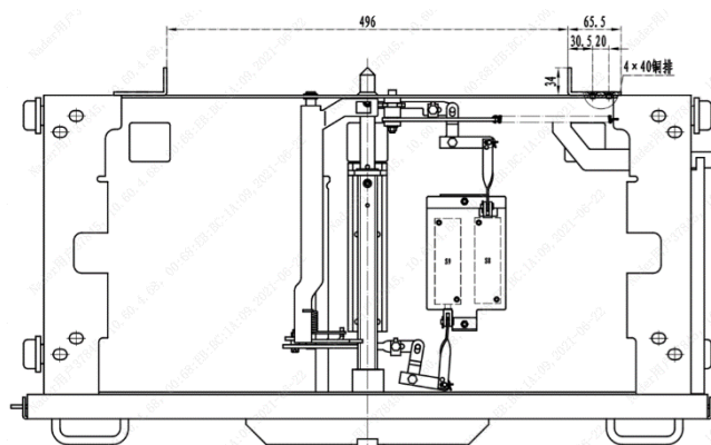
配柜宽 1000mm
