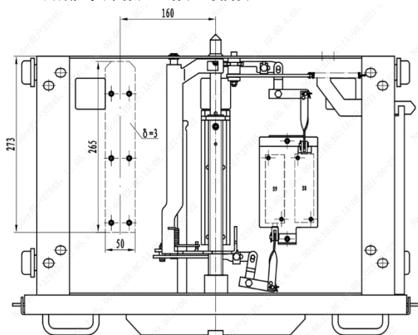
配柜宽 800mm
